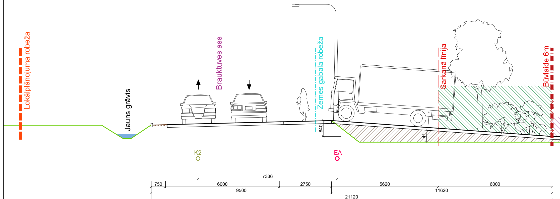
ŠĶĒRSPROFILA GRIEZUMS 1-1 M1:100 / FRAGMENTS F1
