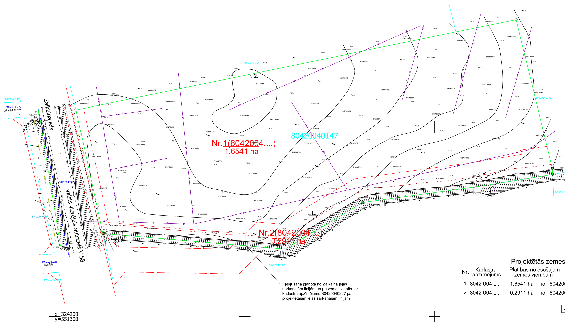
Projektētās teritorijas shēma pirms zemes ierīcības projekta izstrādes
